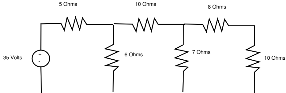
Figure 1: Circuito eléctrico que puede ser descrito por un sistema de ecuaciones lineales
