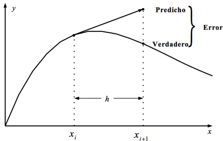
Figure 1: Primera derivada para la estimación de una pendiente.
