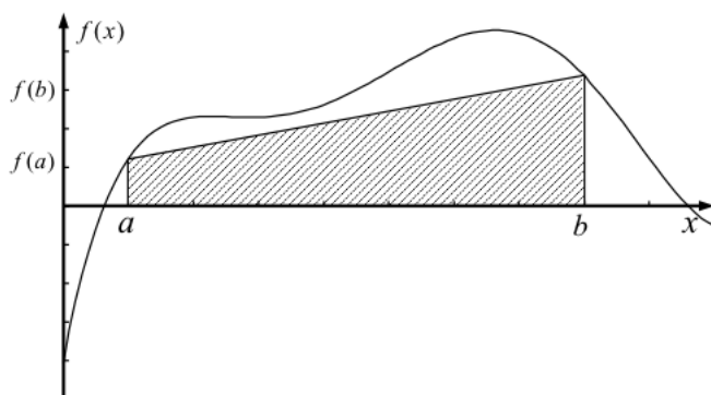
Figure 1: Método de la regla del trapecio.
