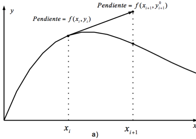
Figure 2: Esquema gráfico del método de Heun. a) Predictor.
