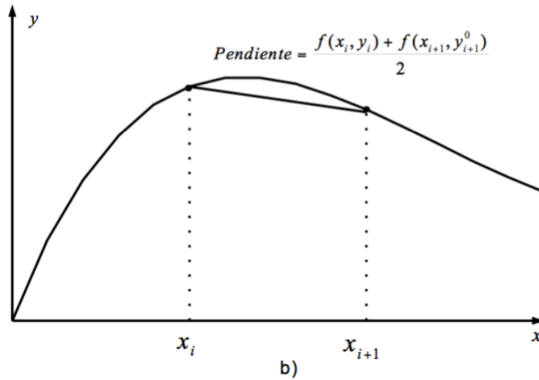
Figure 3: Esquema gráfico del método de Heun. b) Corrector.
